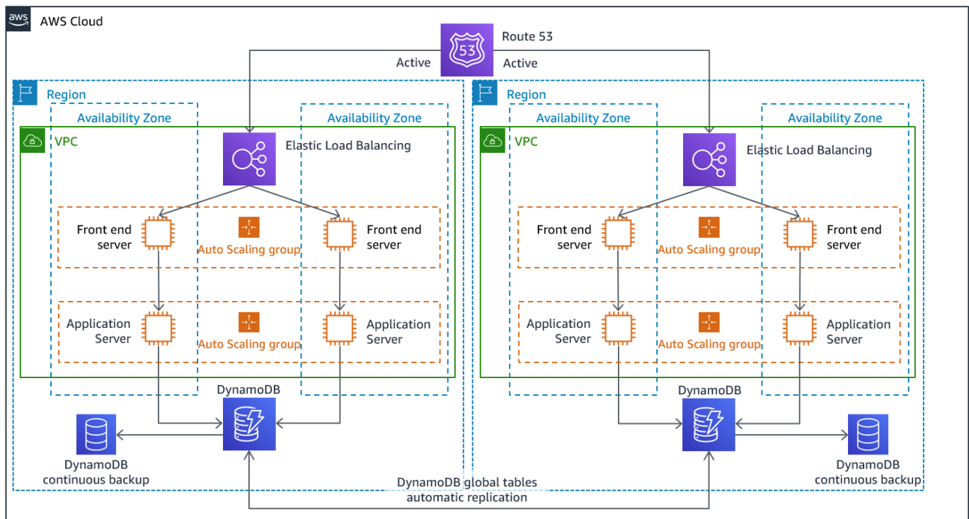
圖 12 - 多站點作用中/作用中架構（將一個作用中路徑變更為非作用中以進行熱待命）
