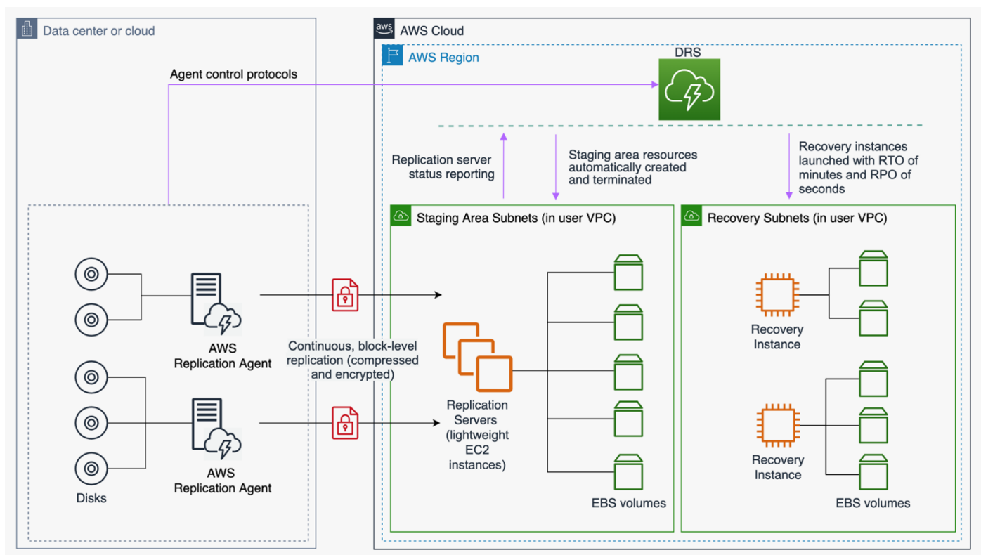
圖 10 - AWS 彈性災難復原架構
