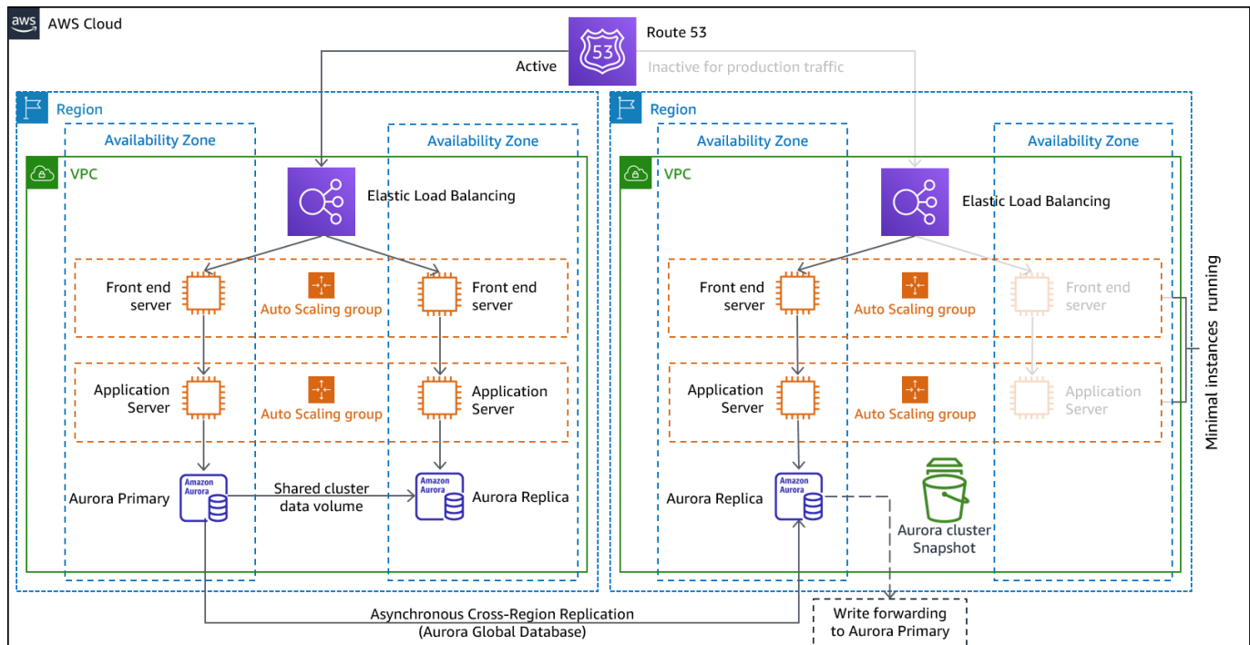
圖 11 - 暖待命架構
