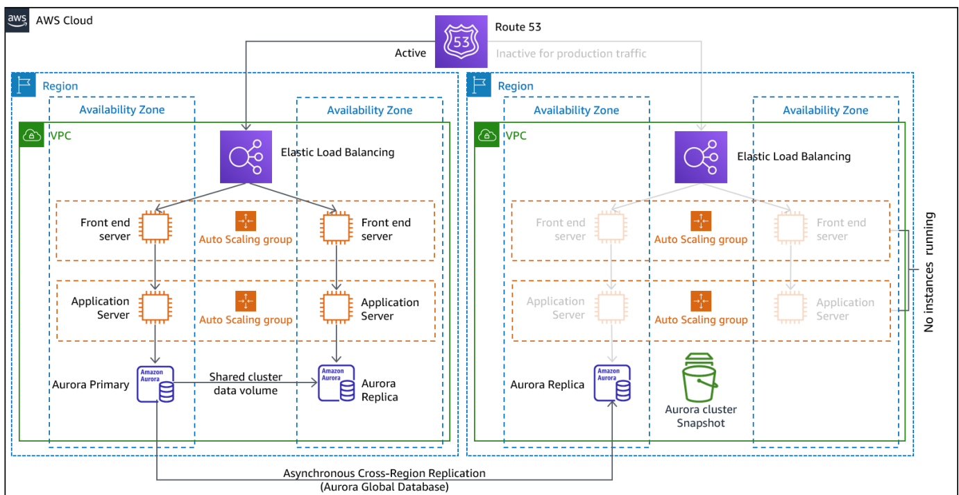
圖 9 - 指示燈架構
