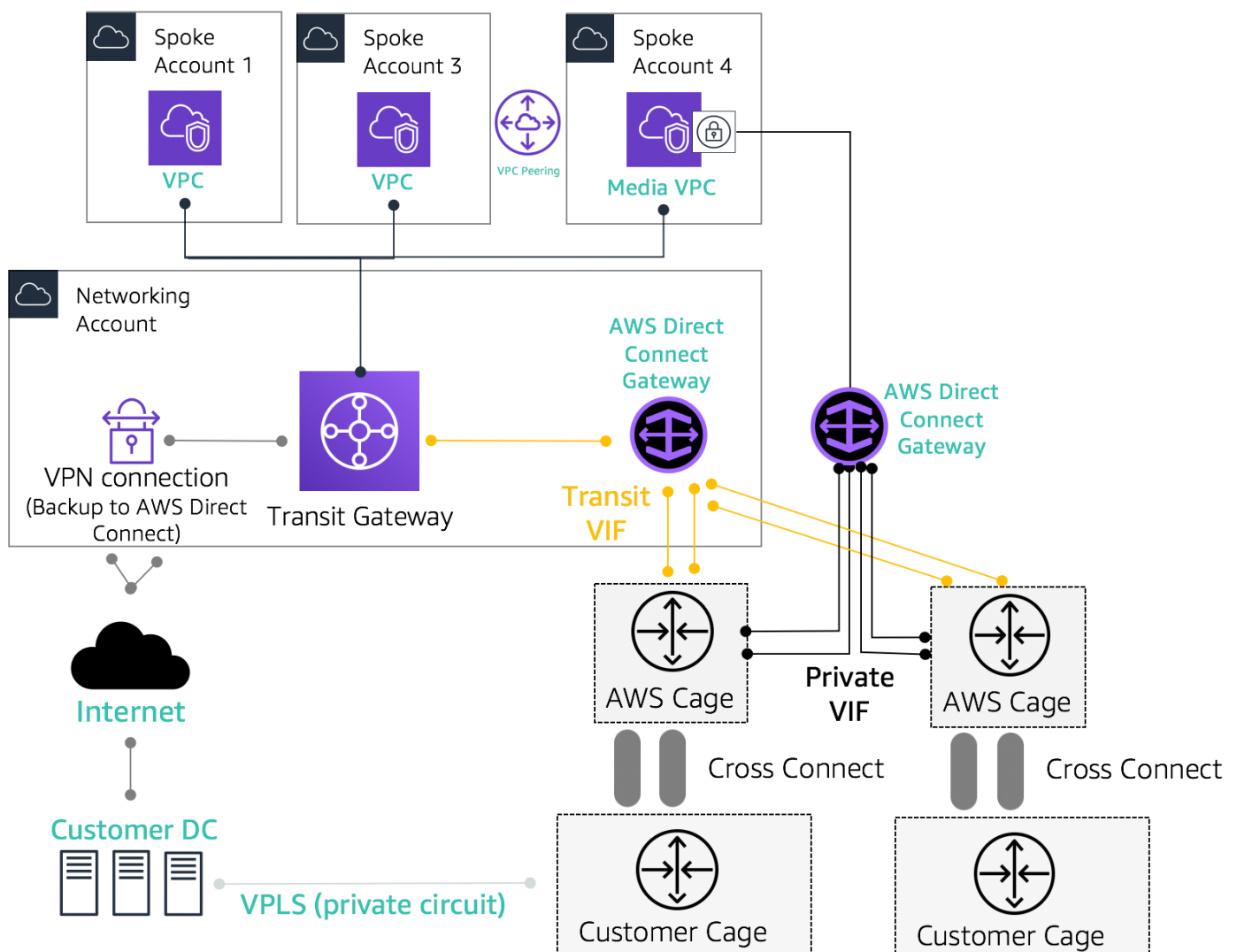
混合連線的範例參考架構
