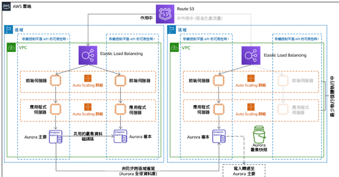
圖 21：暖待命架構
