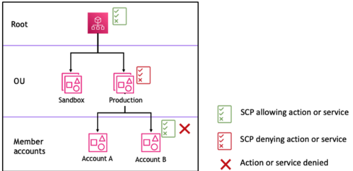
圖 3：在生產 OU 中連接 Deny 陳述式的範例組織結構及其對帳戶 B 的影響
