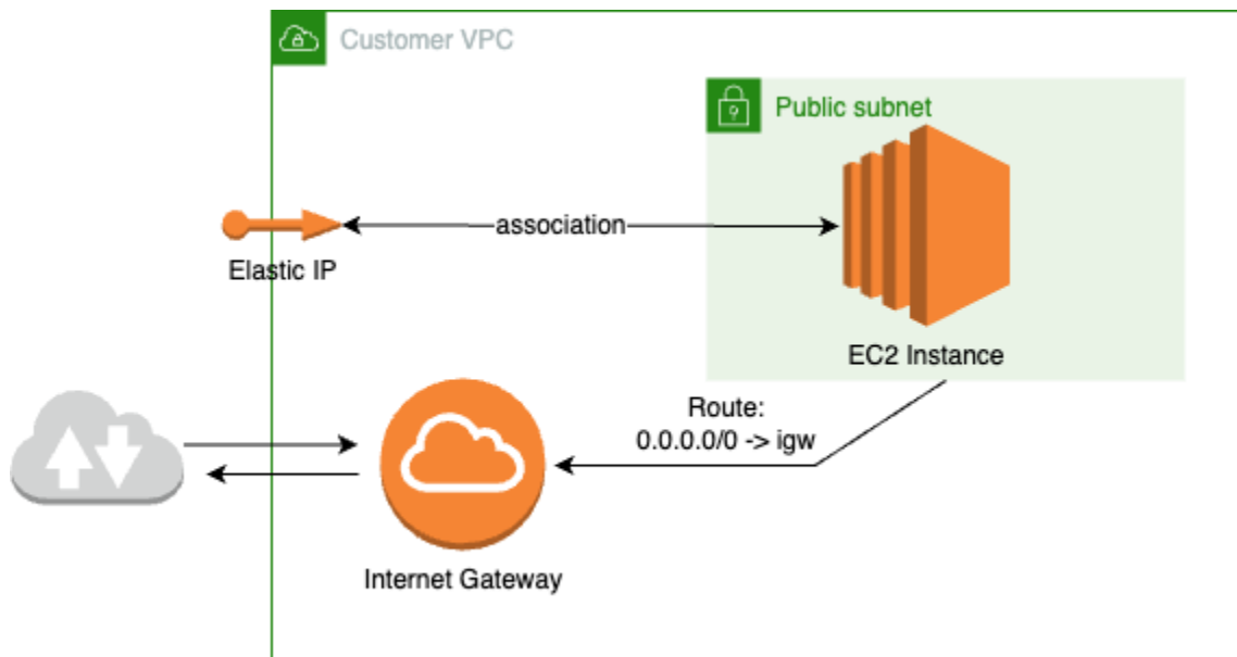
圖表：與公有子網路中的 ENI 相關聯的彈性 IP，連接至私有子網路中的 EC2 執行個體
