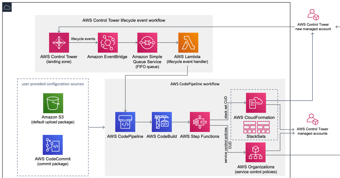
圖 1：AWS Control Tower 架構的自訂
