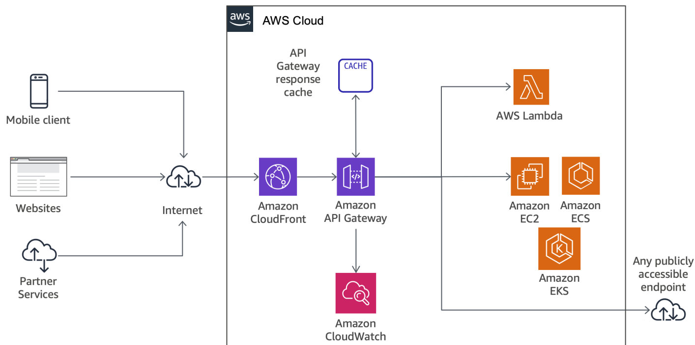
图 3 : API Gateway 调用流程
