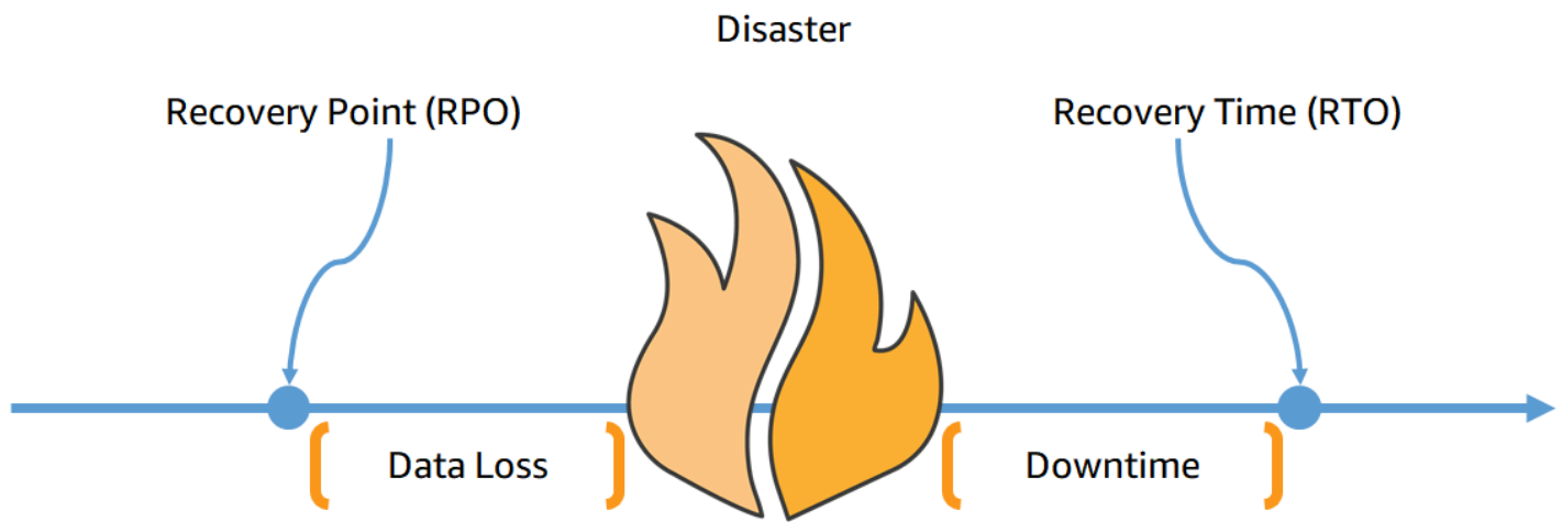
图 3-恢复目标
