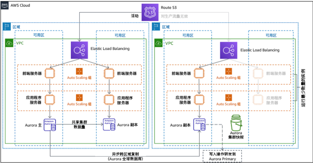
图 21：热备用架构
