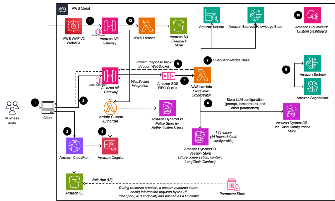
描绘文本用例架构 ( 在禁用 VPC 选项的情况下部署时 )
