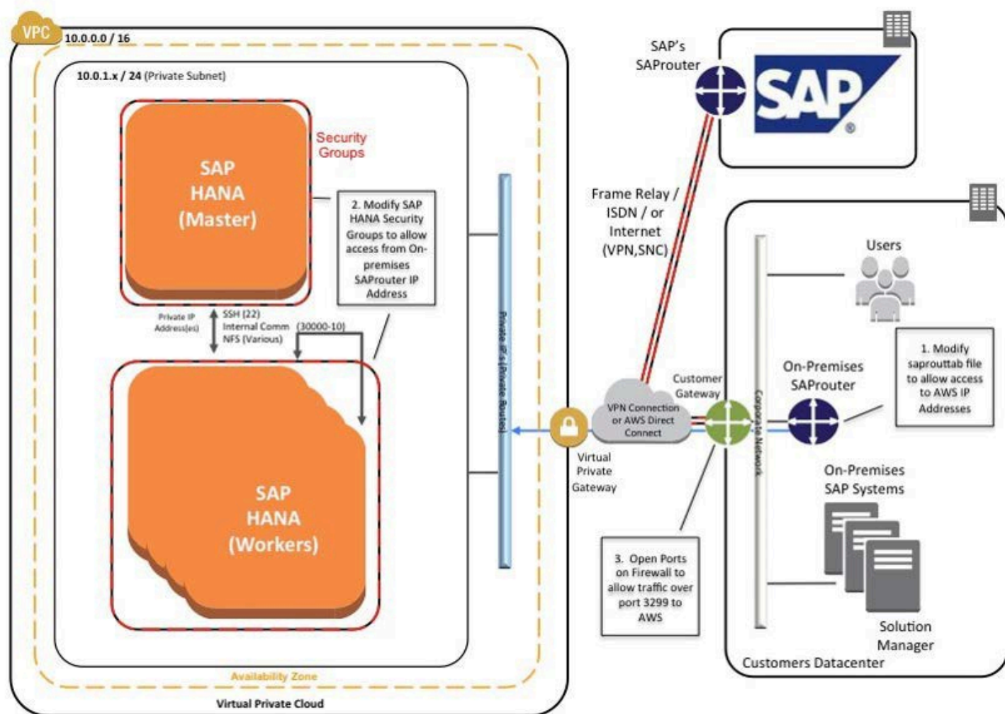
图 14：与内部部署的 Supp SAprouter ort 连接
