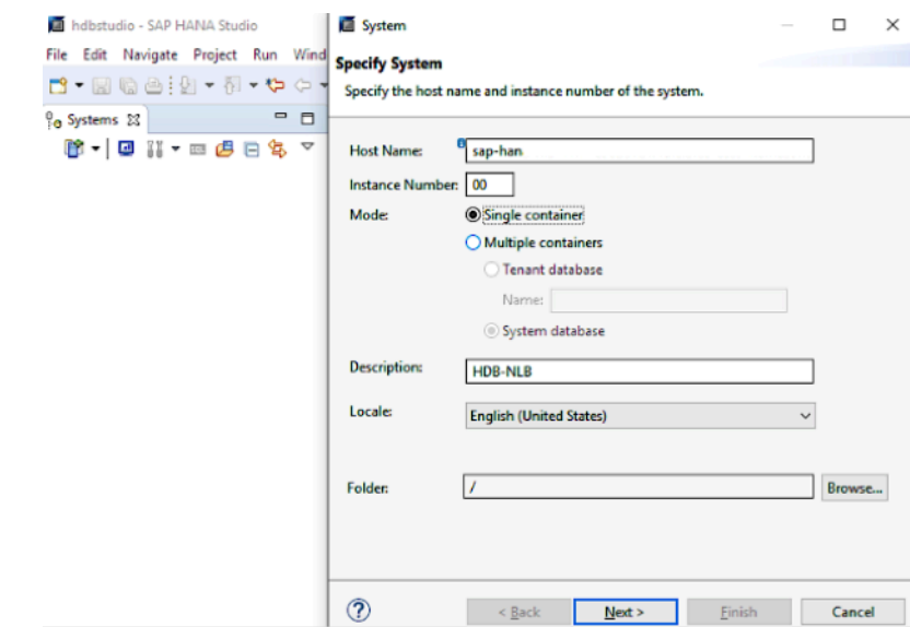
图 10：SAP HANA Studio 中更新的主机名
