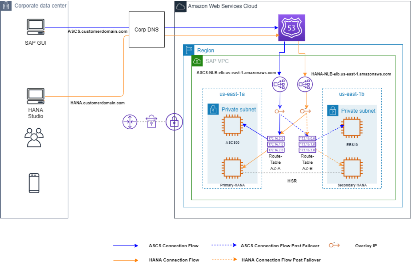
图 6：使用叠加 IP 和 Elastic Load Balancer 实现的 SAP 高可用性
