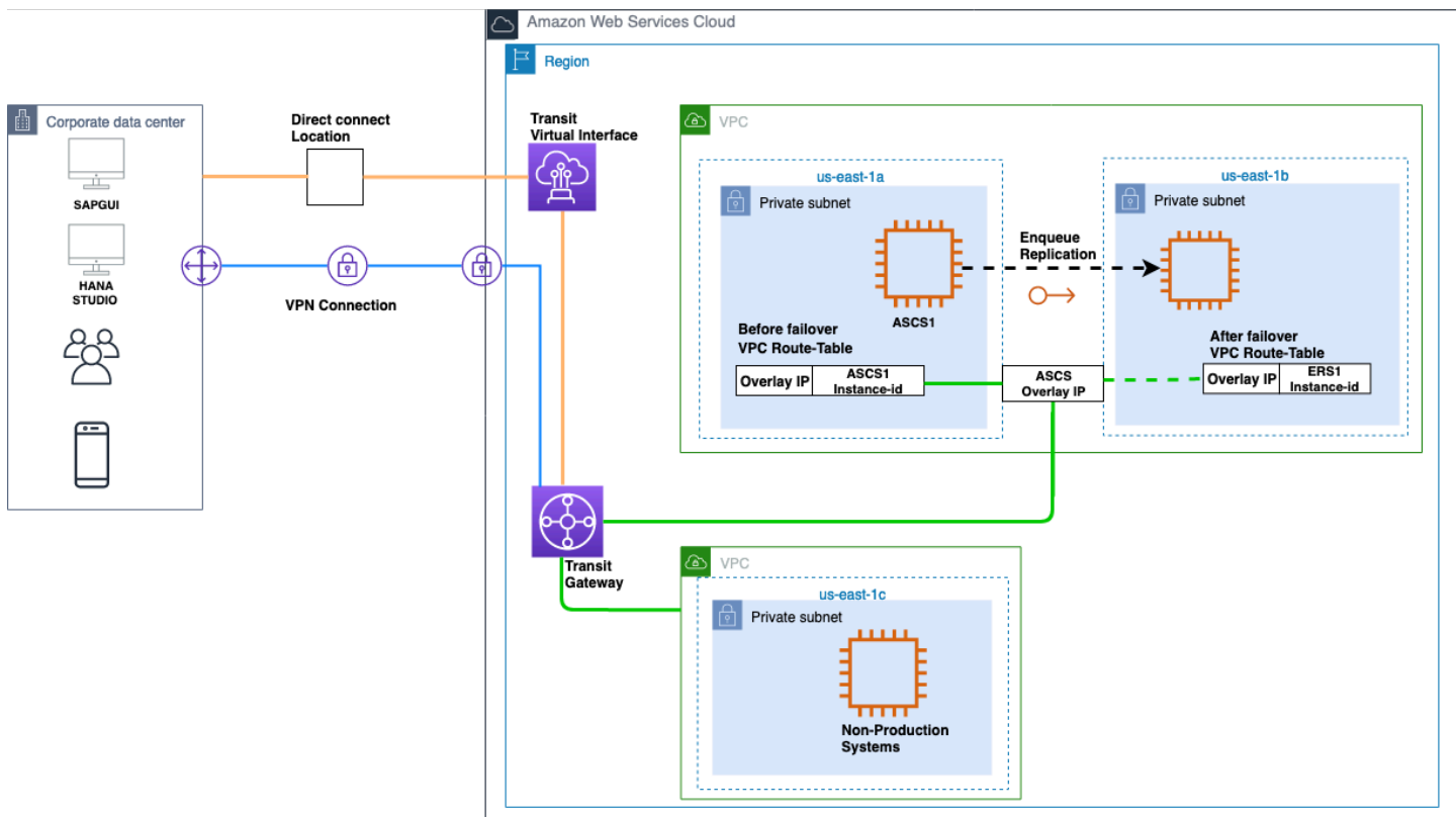
图 1：使用 T AWS ransit Gateway 设置叠加 IP 地址
