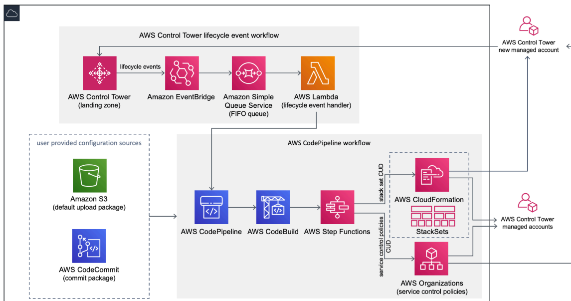
图 1：AWS Control Tower 自定义项的架构
