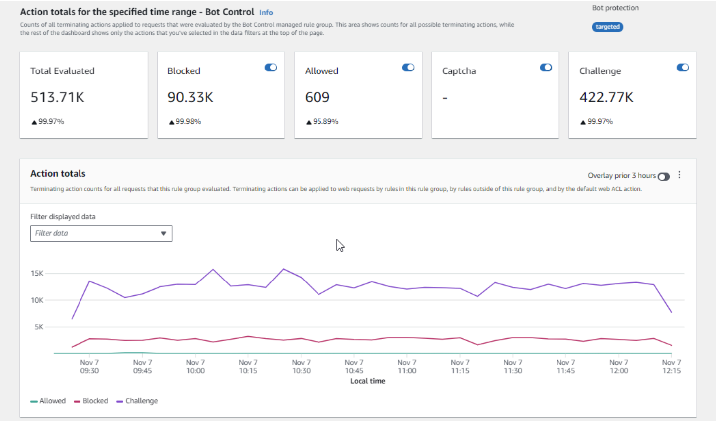
Tela de exemplo: contagem de ações do painel AI Traffic Analysis
