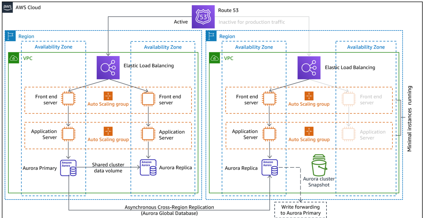
그림 11 - 웜 스탠바이 아키텍처
