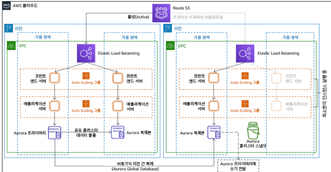
그림 21: 웜 대기 아키텍처
