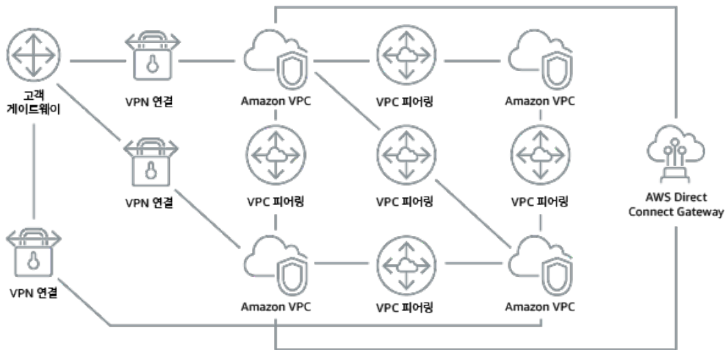
그림 1: AWS Transit Gateway가 없는 경우: VPN 연결을 사용하여 각 Amazon VPC를 서로 피어링하고 각 온사이트 위치에 피어링해야 합니다. 이 경우 확장에 따라 복잡성이 증가할 수 있습니다.
