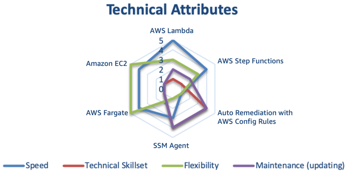
図 4: 自動対応アプローチ間の技術属性の違い
