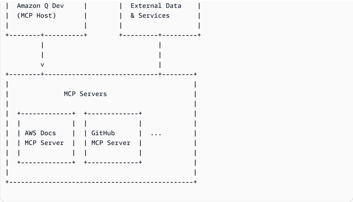
<caption> Amazon Q Developer CLI が MCP サーバーを介して外部データソースに接続する方法を示す MCP アーキテクチャ </caption>
