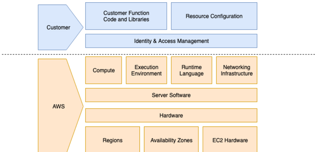
Gambar 1 - Model tanggung jawab bersama untuk AWS Lambda
