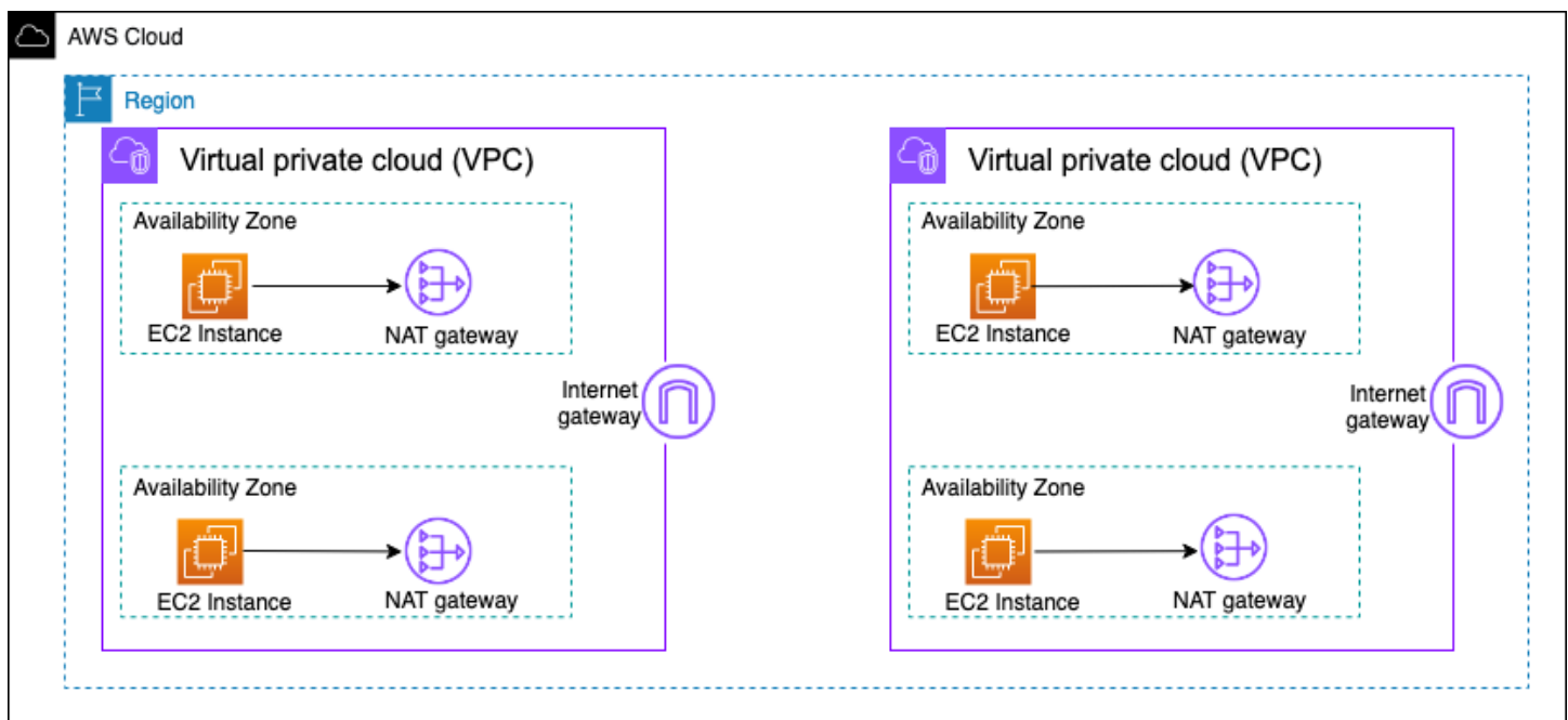
Architecture de passerelle NAT à haute disponibilité décentralisée
