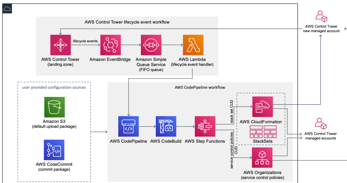
Figure 1 : Personnalisation pour l'architecture AWS Control Tower
