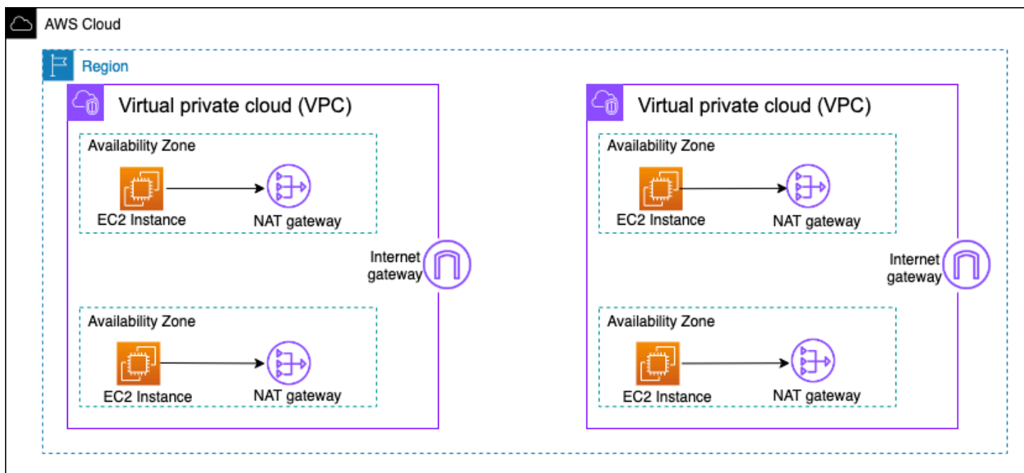
Arquitectura de puerta de enlace NAT descentralizada de alta disponibilidad
