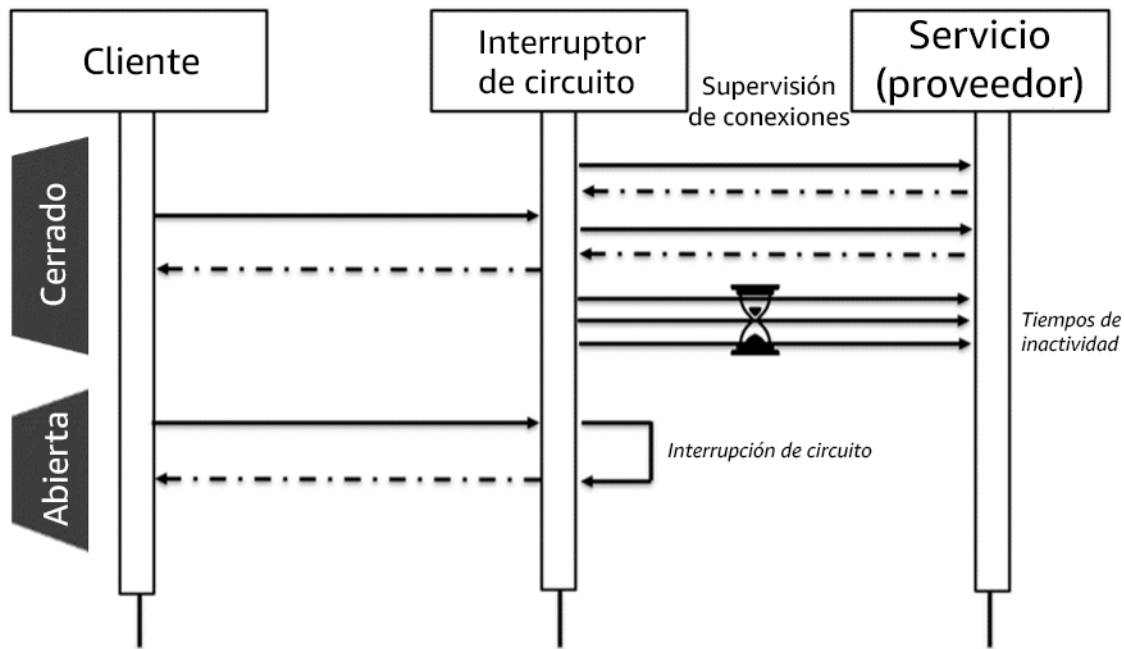
Figura 6: Disyuntor que muestra los estados abierto y cerrado.
