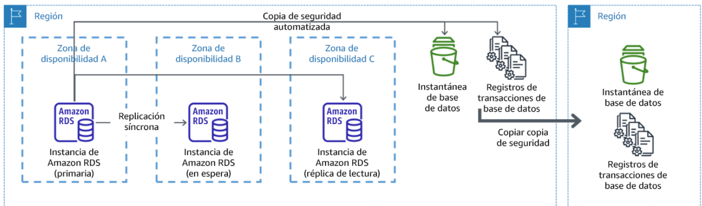
Figura 10: Un despliegue de base de datos multi-AZ resiliente con copia de seguridad en otra región de AWS
