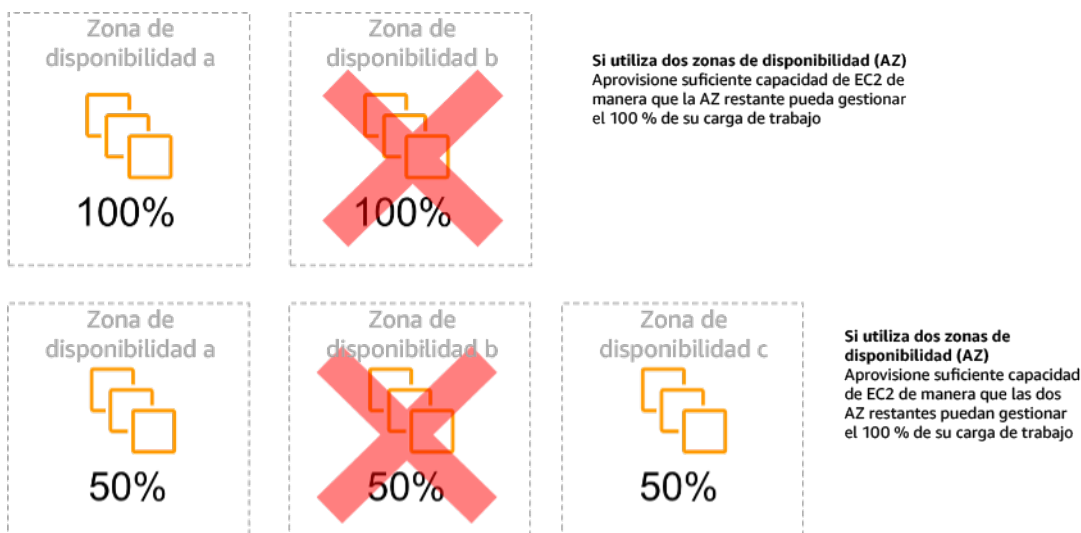
Figura 14: Estabilidad estática de las instancias EC2 entre zonas de disponibilidad
