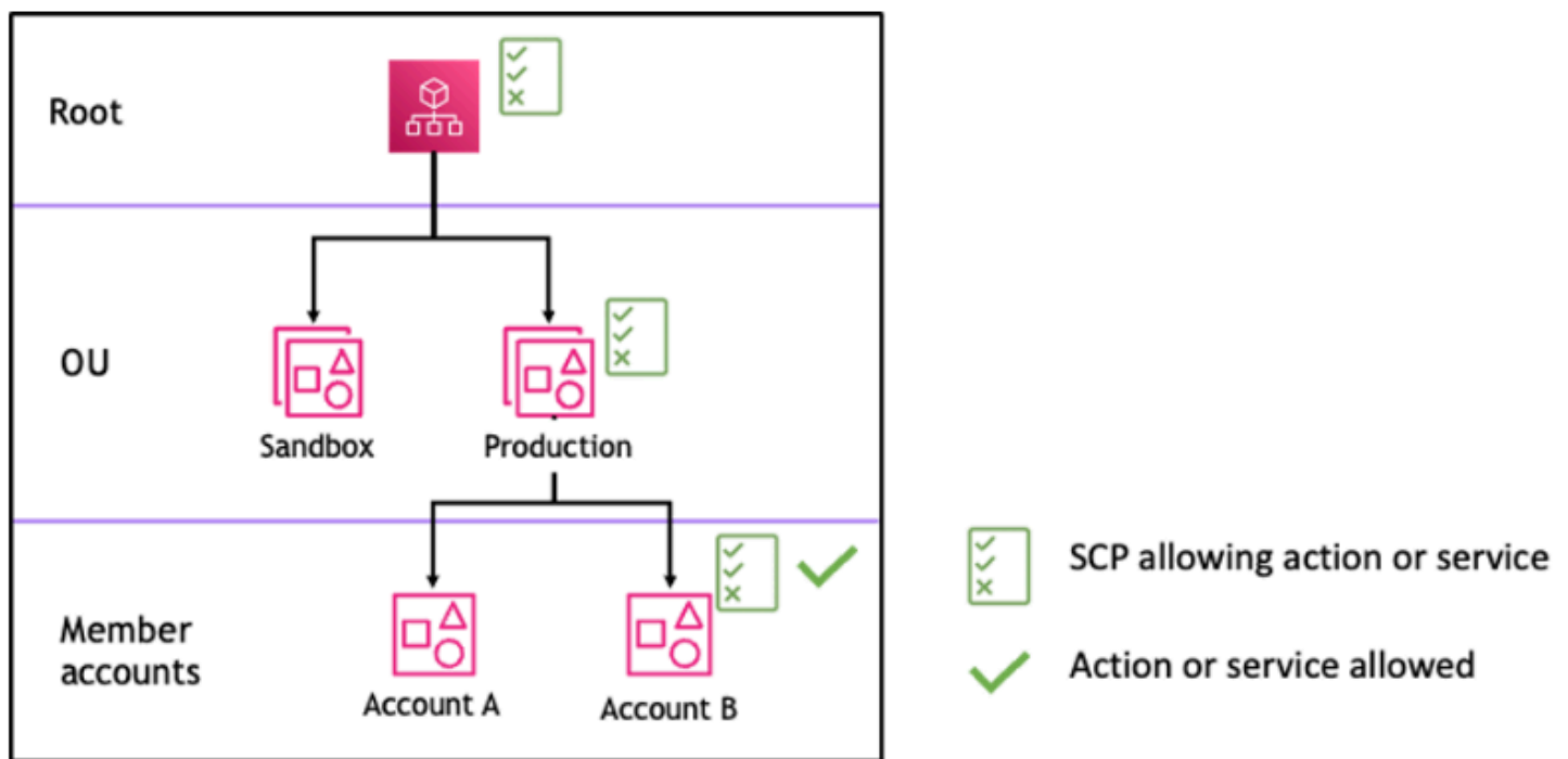
Abbildung 1: Beispiel für eine Organisationsstruktur mit einer Allow Erklärung, die an Root, Production OU und Account B angehängt ist
